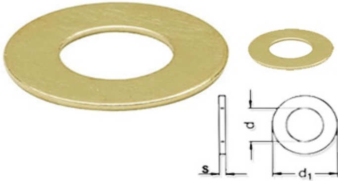
DIN 125 Brass Washers Brass Flat Washers DIN 125
