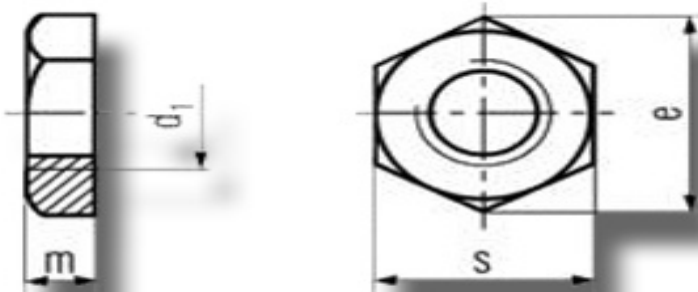
DIN 431 Brass Jam Nuts
