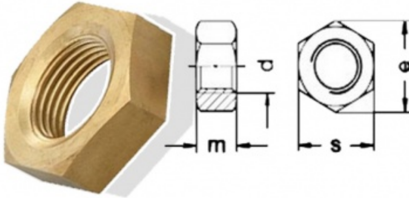
DIN 934 Brass hex nuts
