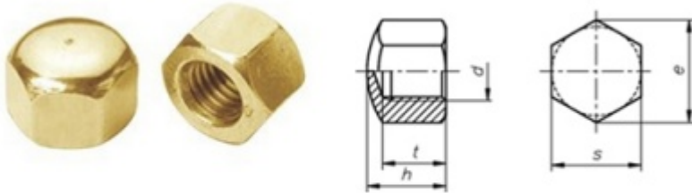
BRASS HEX CAP NUTS DIN 917 BRASS NUTS
